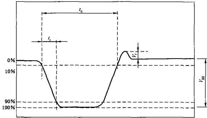
a) 方波脉冲
