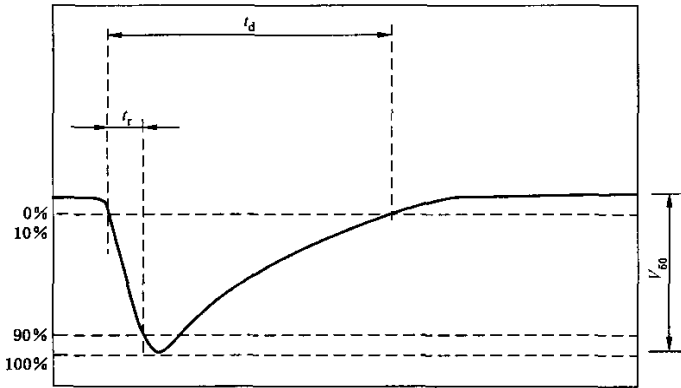
b) 尖峰脉冲
