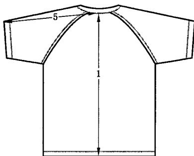
b) 短袖上衣主要部位规格尺寸的测量部位
