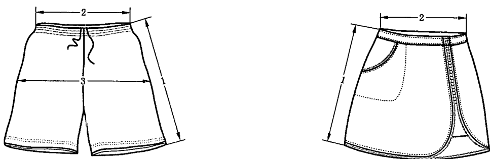
a) 短裤主要部位规格尺寸的测量部位 b) 裙子主要部位规格尺寸的测量部位 1——裤(裙)长; 2——1/2 腰围; 3——1/2 臀围。
