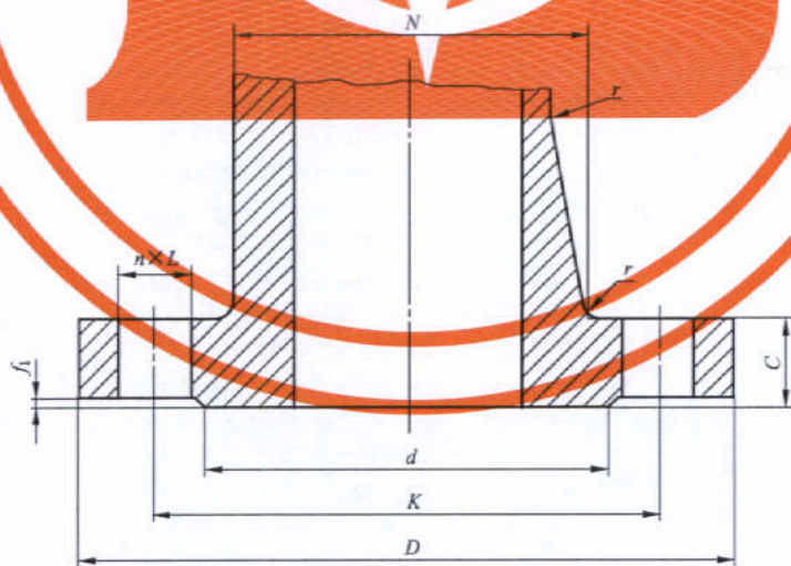
图 2 突面 (RF) 整体钢制管法兰 (适用于 PN 2.5、PN 6、PN 10、PN 16、PN 25、PN 40、PN 63、PN 100、PN 160、PN 250、PN 320 和 PN 400)
