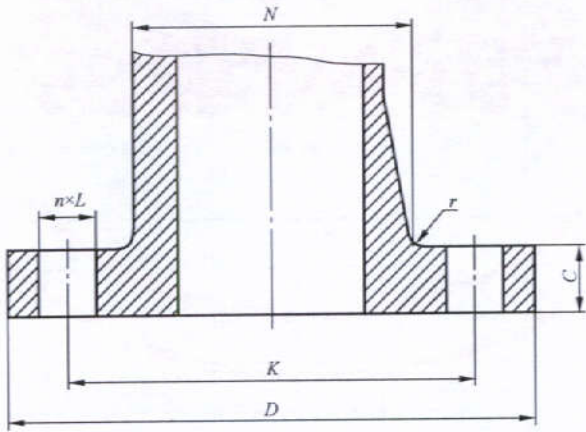
图 7 平面(FF)整体钢制管法兰 (适用于 Class 150)
