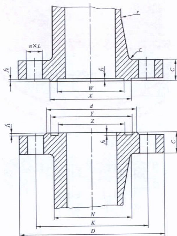
图 4 榫槽面(TG)整体钢制管法兰
