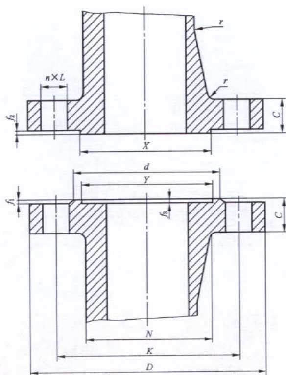
图 3 凹凸面(MF)整体钢制管法兰
