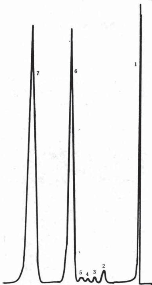
五氯硝基苯粉剂色谱图
