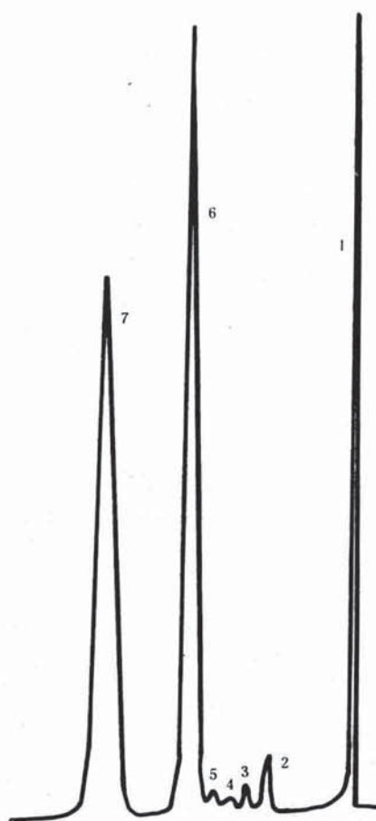
五氯硝基苯粉剂色谱图
