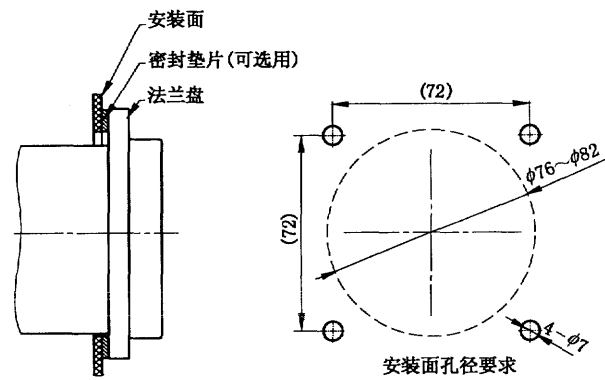
图 C.1 车辆插座前安装方式安装示例
