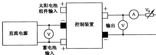
图5 放电回路压降测试电路
