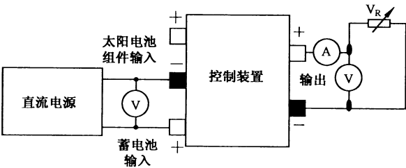
图 3 欠压断开和恢复功能测试电路
