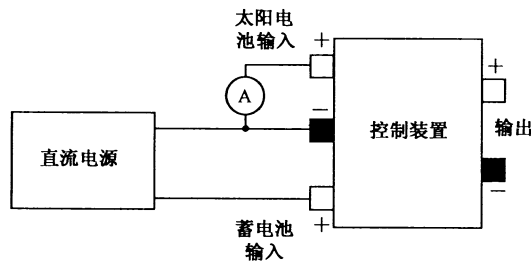
图7 蓄电池反向放电保护功能测试电路
