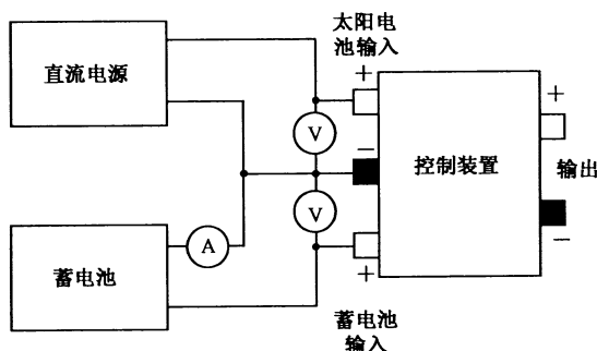
图6 充电回路压降测试电路
