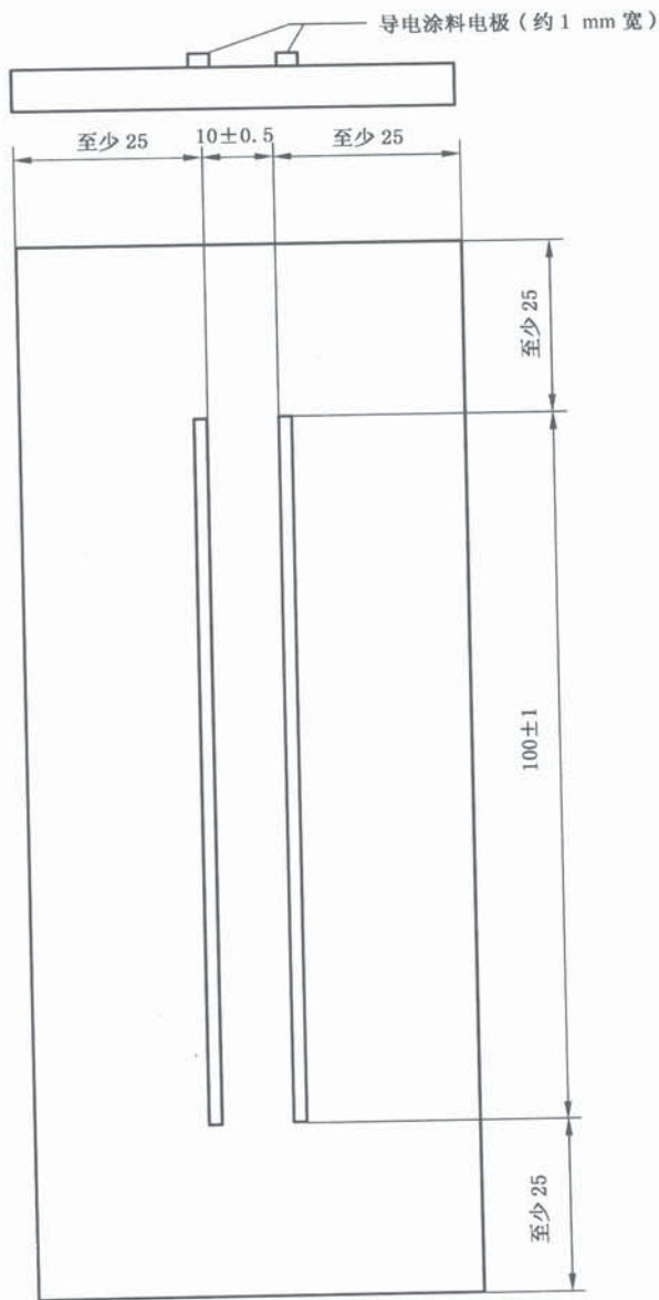
图 A.1 带导电涂料电极的板状试样
