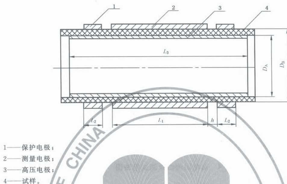
图2 管状试样电极配置
