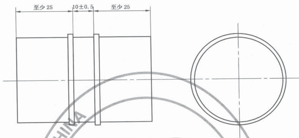
图 A.2 带导电涂层的管和棒状试样
