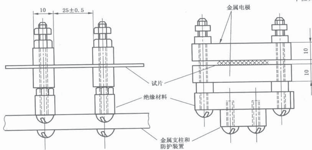
图 A.4 用于条形材料的电极
