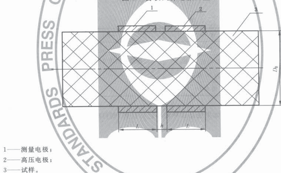
图3 棒状试样电极配置
