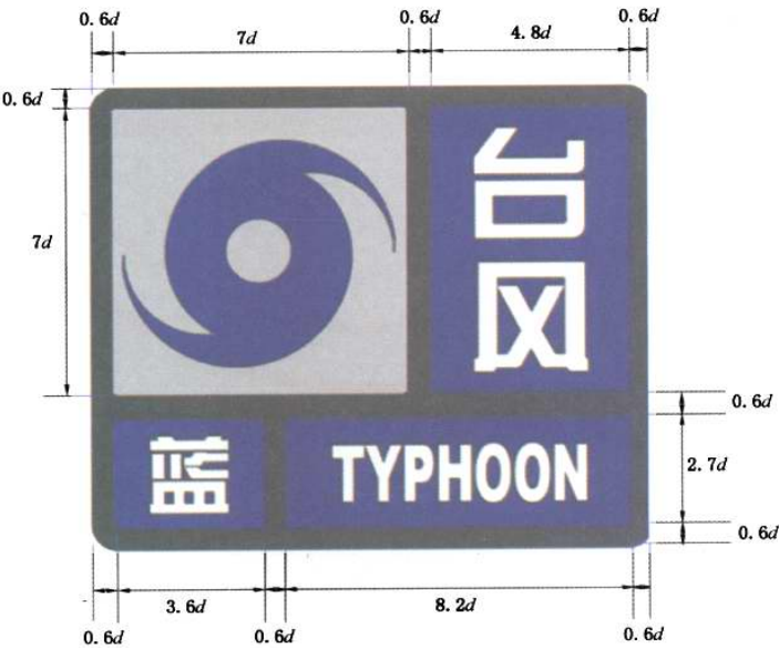
图 A.1 气象灾害预警信号图标的设计要求
