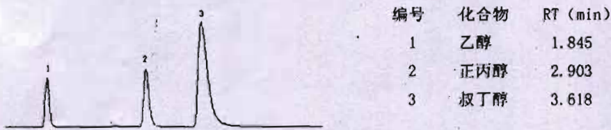
图A. 2 PLOT Q毛细管柱血中酒精含量检测色谱图 (柱2)
