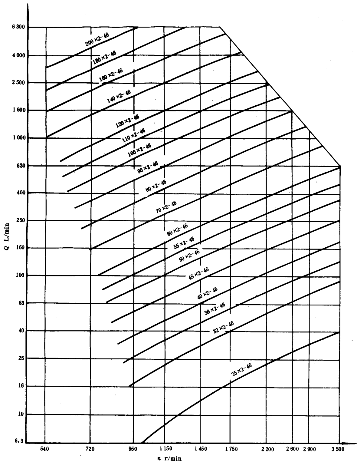
图 2 单吸、2个螺距泵型谱
