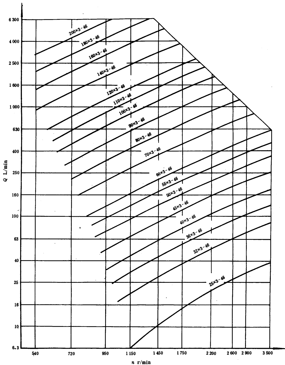
图 4 单吸、3个螺距泵型谱
