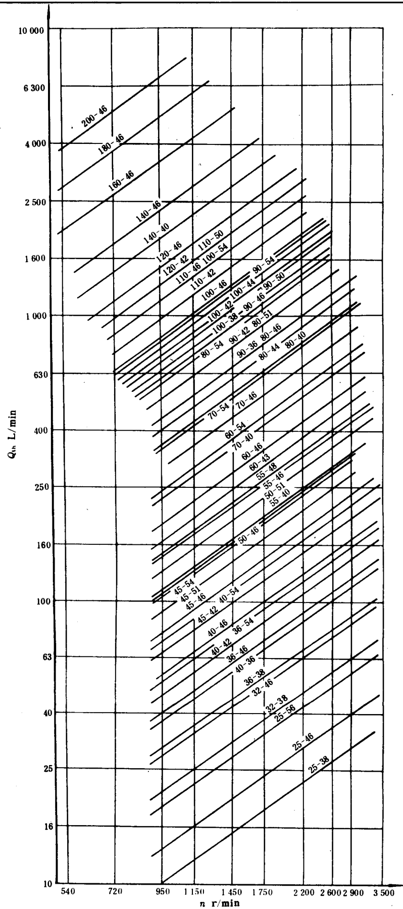
图 A1 单吸泵理论流量型谱
