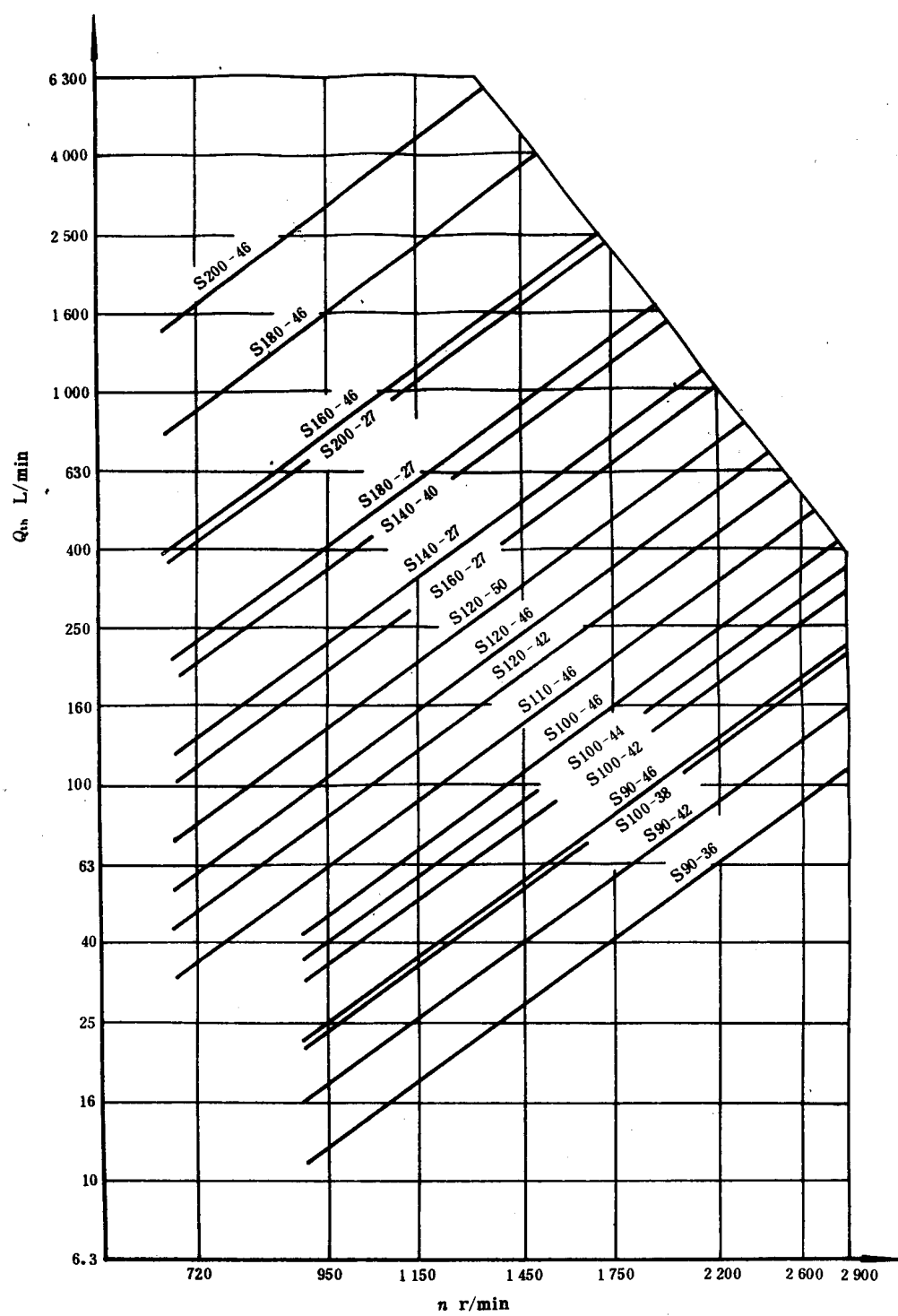
图 A2 双吸泵理论流量型谱
