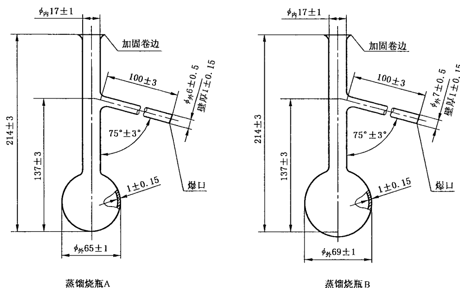
图 A.1 蒸馏烧瓶 A(100 mL)、蒸馏烧瓶 B(125 mL)
