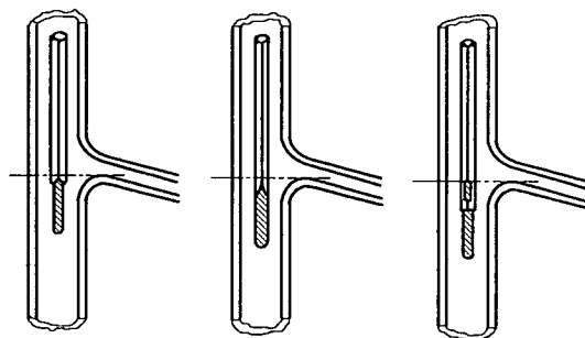
图 4 温度计在蒸馏烧瓶中的位置
