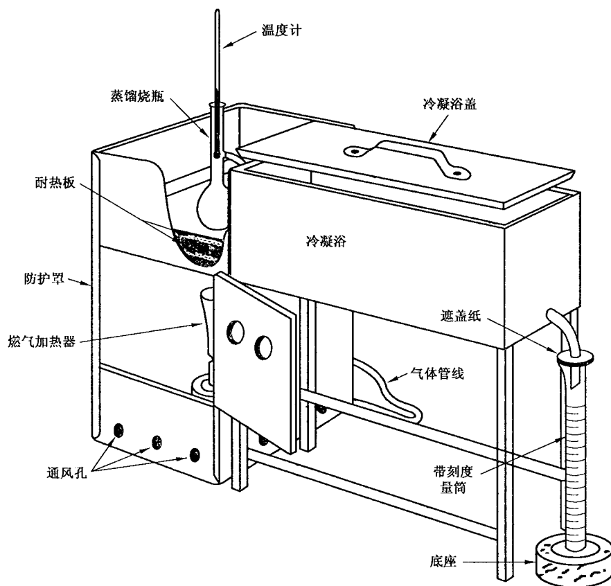
图 1 燃气加热型蒸馏仪器装置图
