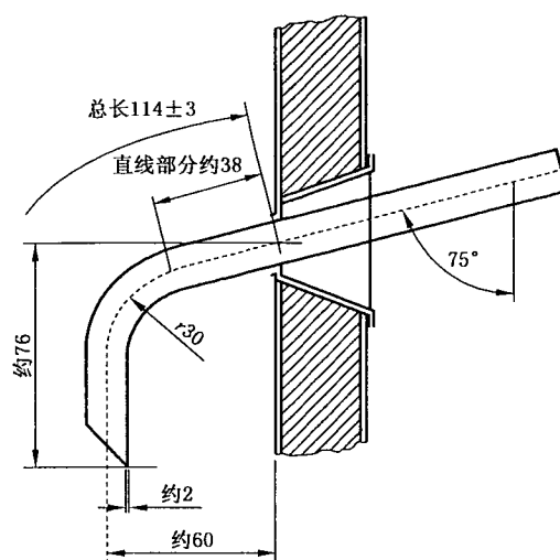
图 A.2 冷凝管下部结构图
