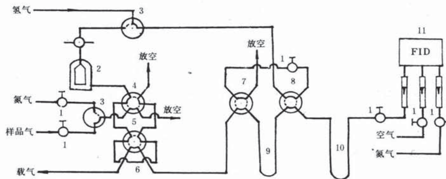
图 A2 转化氢焰色谱切割气路示意图
