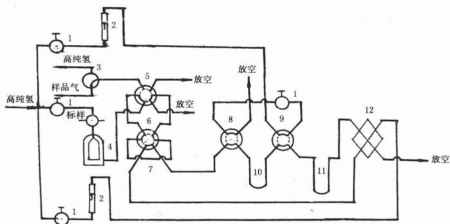
附录 A 气路流程和冻结器结构示意图 (参考件)
