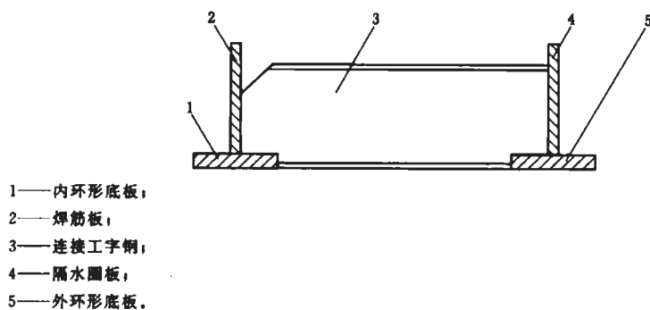
图 4 梁板式法兰盘截面
