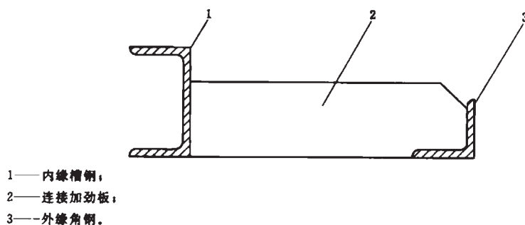
图 3 型钢法兰盘截面
