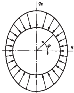
图 1 不均匀荷载变化规律图
