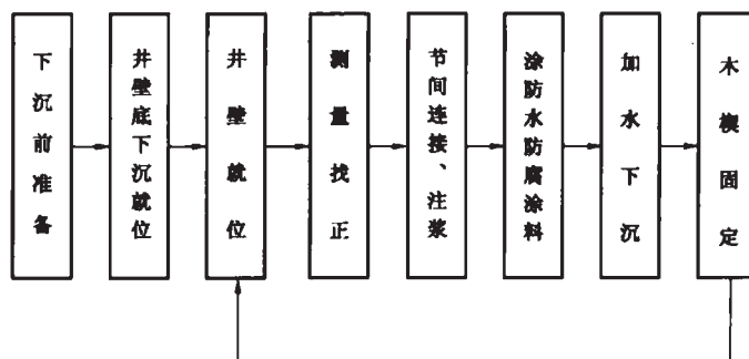
图 5 井壁悬浮下沉工艺流程示意图
