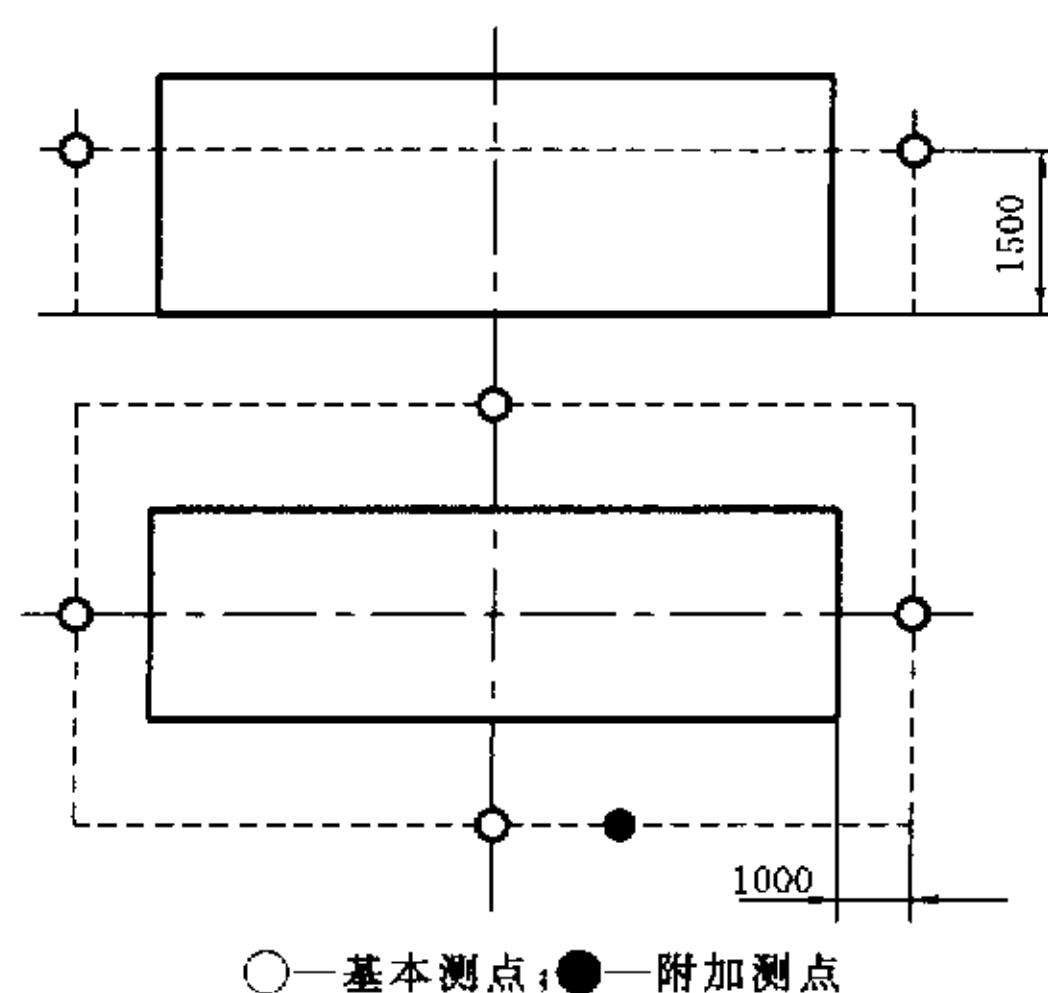
图 1 测点布置图
