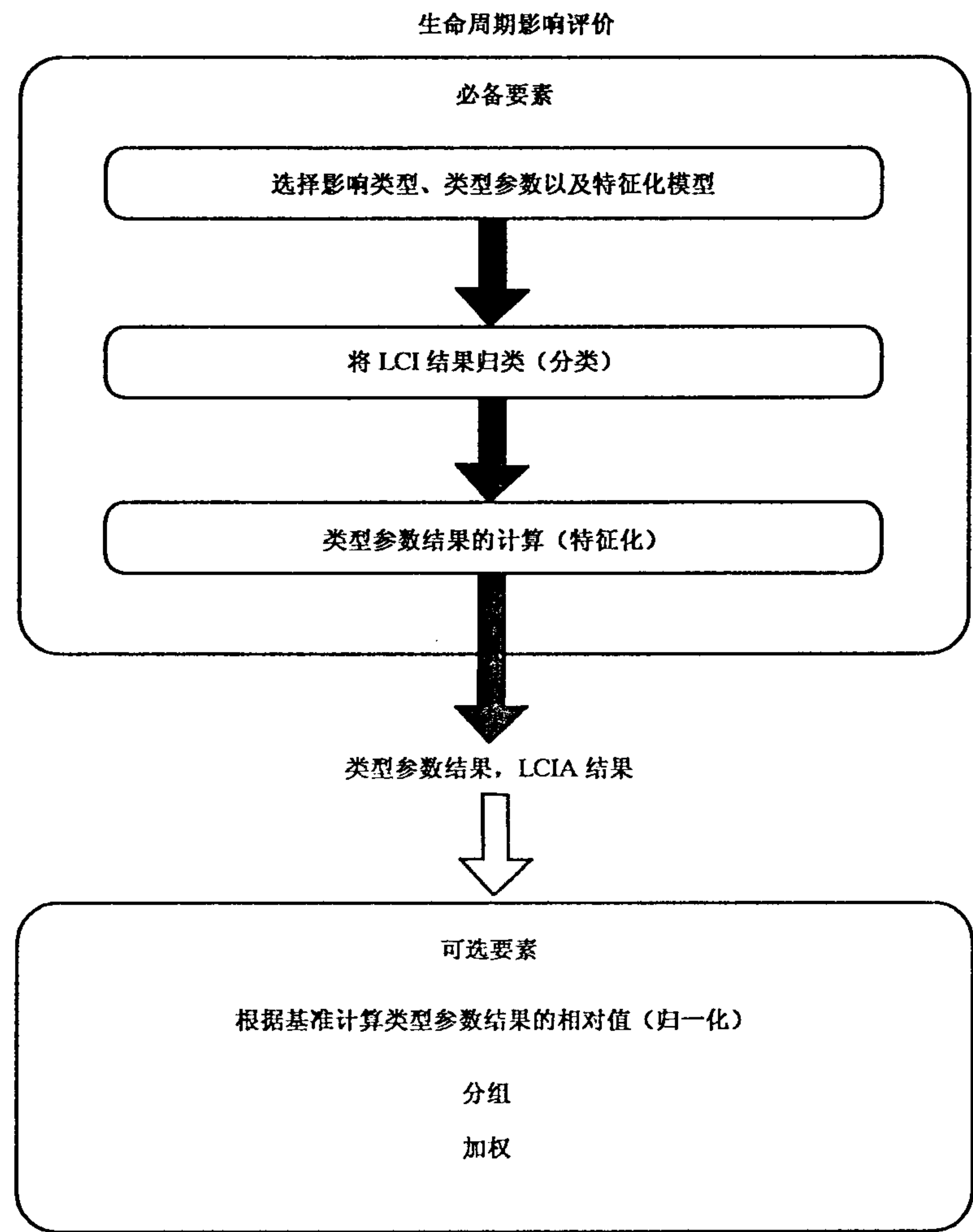
图 4 LCIA 阶段的要素
