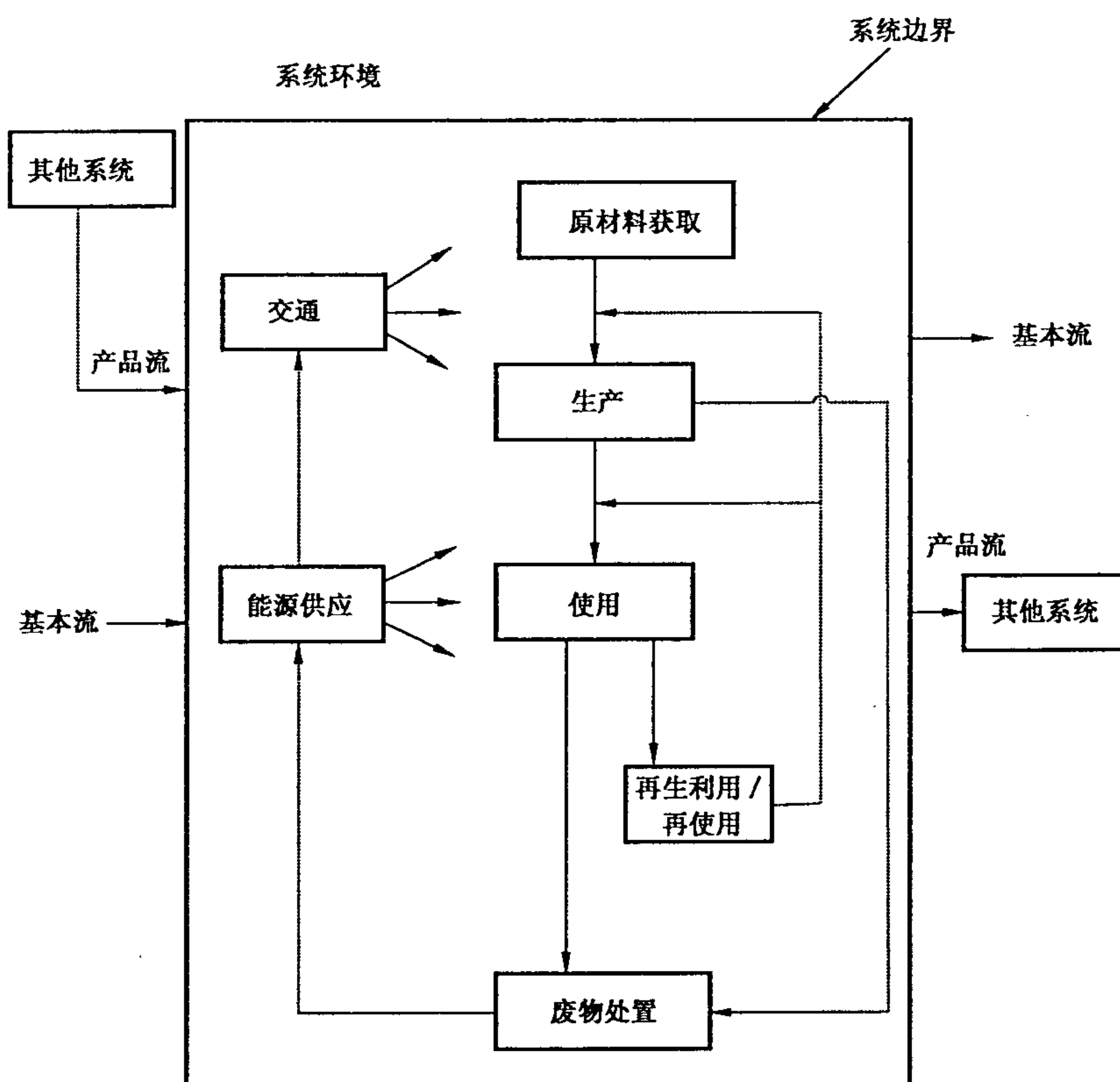
图 2 LCA 中产品系统的示例
