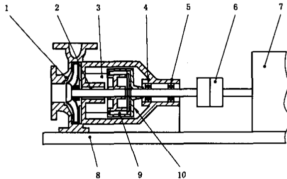
图 1 屏蔽电泵
