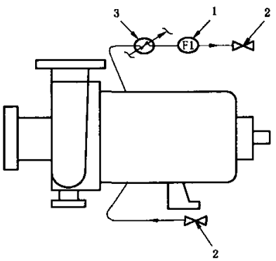
方案P 热交换器的加热或冷却
