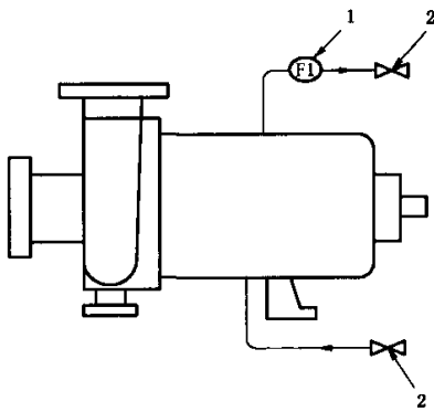
方案A 传动部分的加热或冷却
