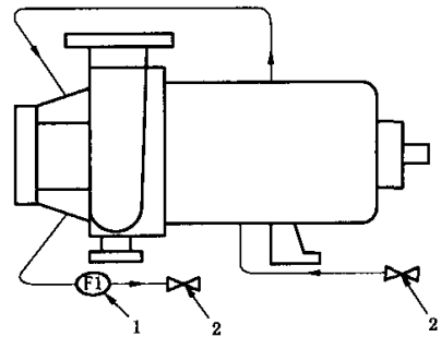
方案N 传动部分和壳体夹套的加热或冷却
