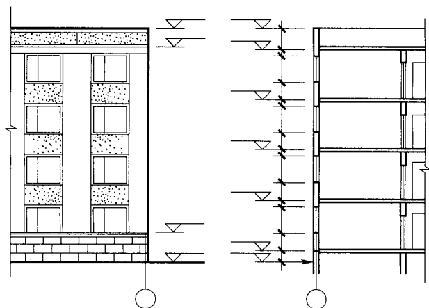
图 4.4.5 相邻立面图、剖面图的位置关系
