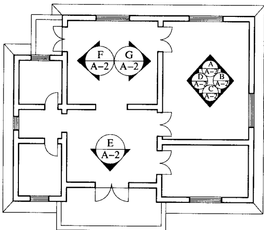
图 4.1.8-3 平面图上内视符号(带索引)应用示例
