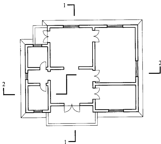
图 4.3.4 剖切符号
