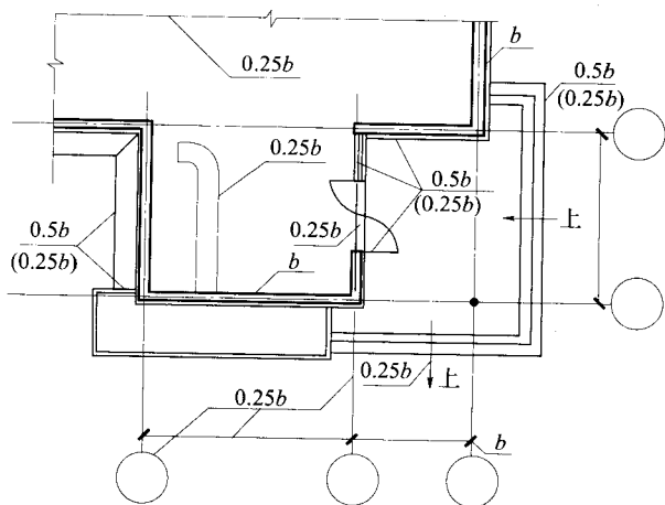
图 2.1.1-1 平面图图线宽度选用示例
