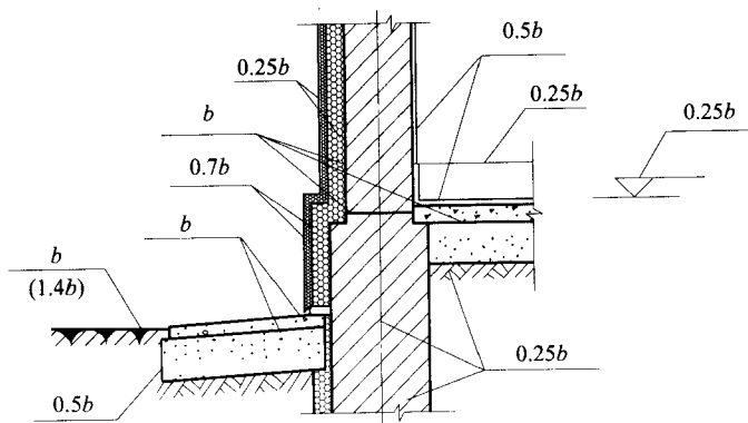
图 2.1.1-2 墙身剖面图图线宽度选用示例
