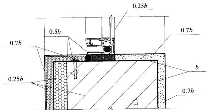
图 2.1.1-3 详图图线宽度选用示例
