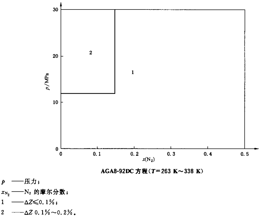
图 E.1 计算高含 N_2 天然气压缩因子时不确定度的估计范围
