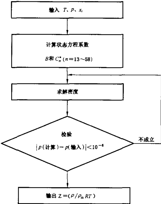
图 B.1 AGA8-92DC 计算方法的程序流程图
