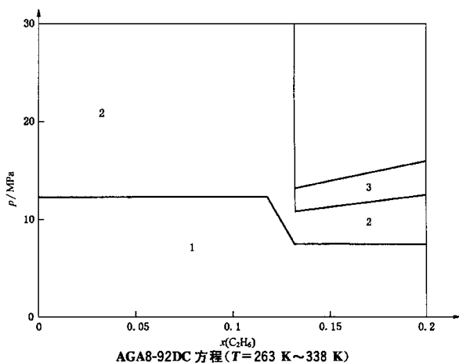
图 E.2 计算高含 \text{CO}_2 天然气压缩因子时不确定度的估计范围
