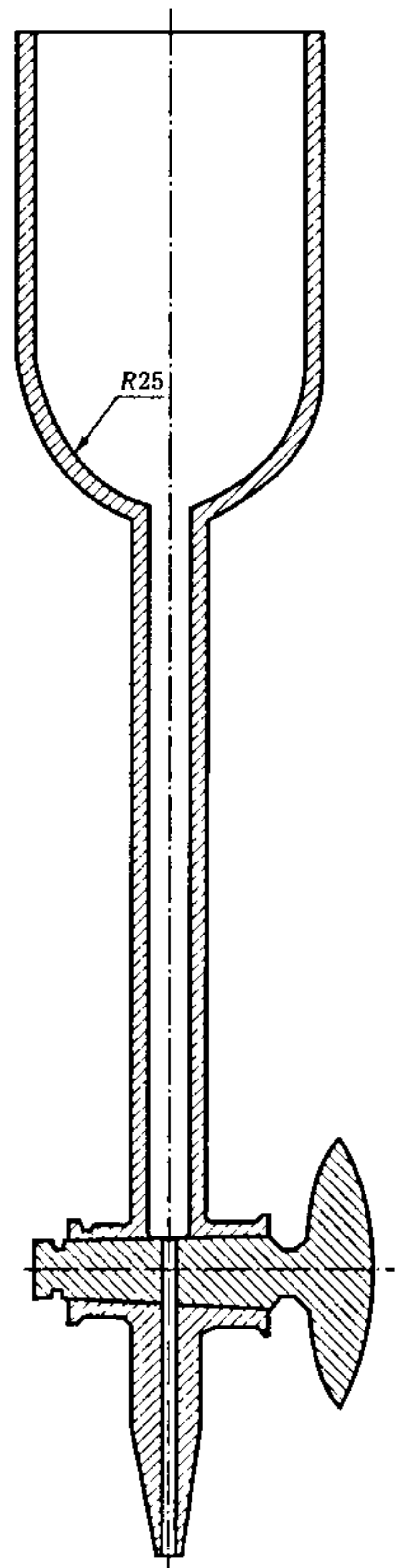
图 A.1 离子交换树脂柱示意图
