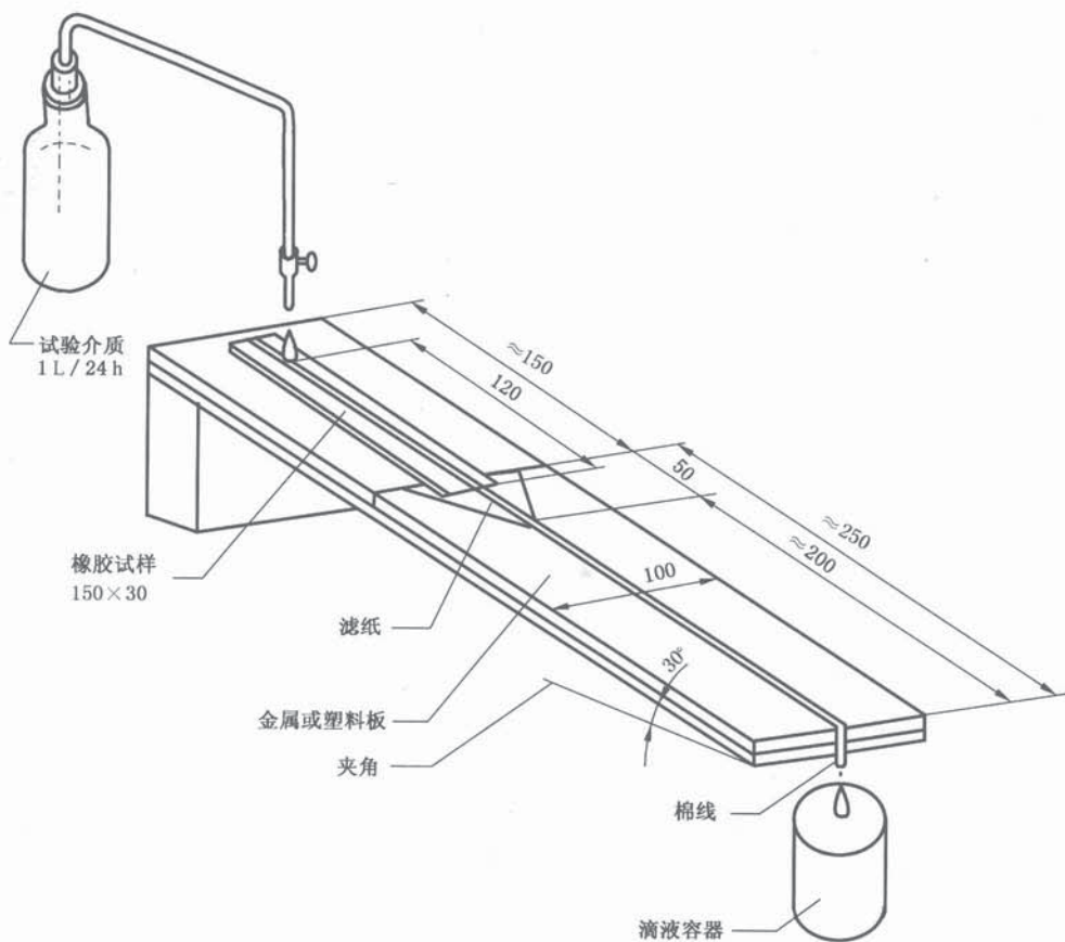
图 1 B1 法滴液装置
