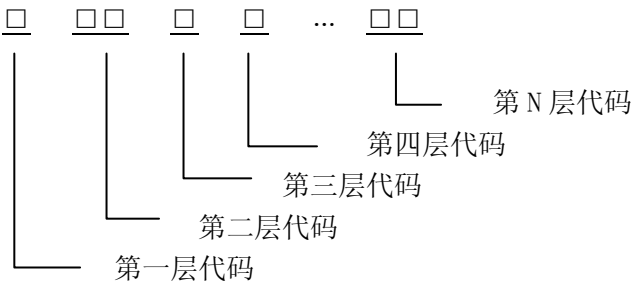
图1 代码结构图
