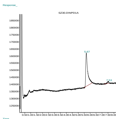
图 D.1 多菌灵气相色谱图
