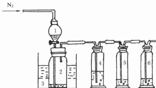
图 1 高锰酸钾吸收装置
