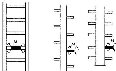
图 B.8 横档扭力试验布置图
