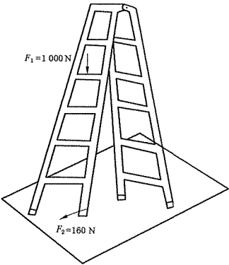
图 B.11 滑移试验
