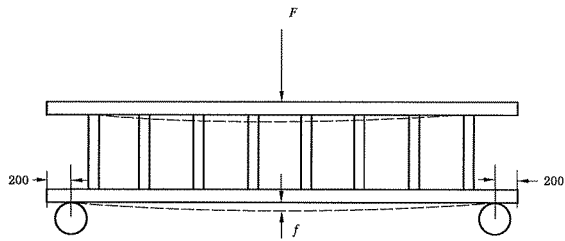
图 B.6 侧面挠度试验布置图
