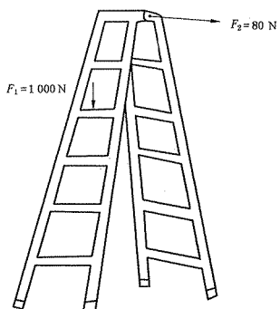
图 B.10 侧稳定试验
