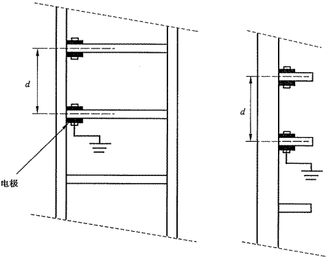
图 B.12 机械老化后电气试验布置图
