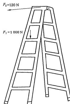
图 B.9 前稳定试验
