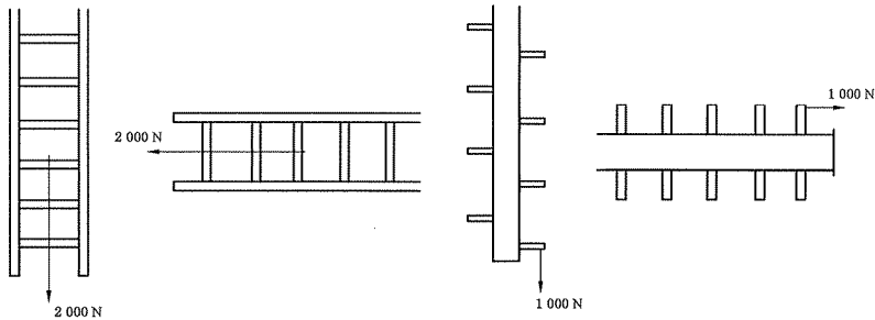
图 B.2 横档强度试验布置图
