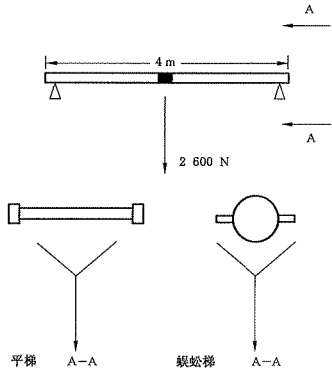
图 B.1 水平强度试验布置图
