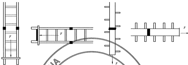
图 B.3 连接装置强度试验布置图
