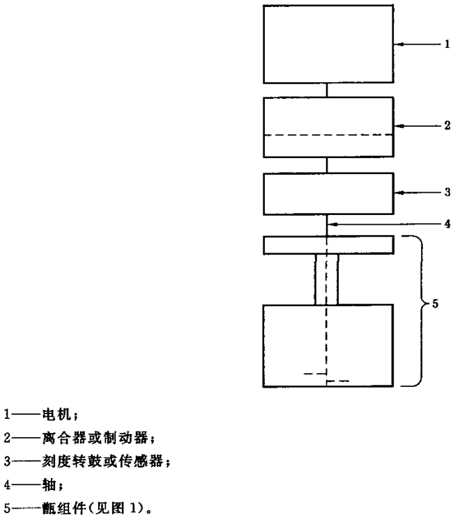
图 3 塑性仪头示意图
