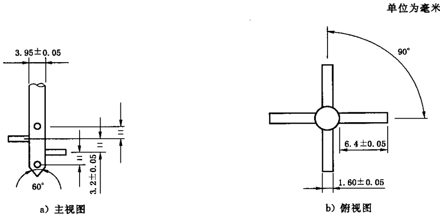
图 2 搅拌桨桨臂示意图
