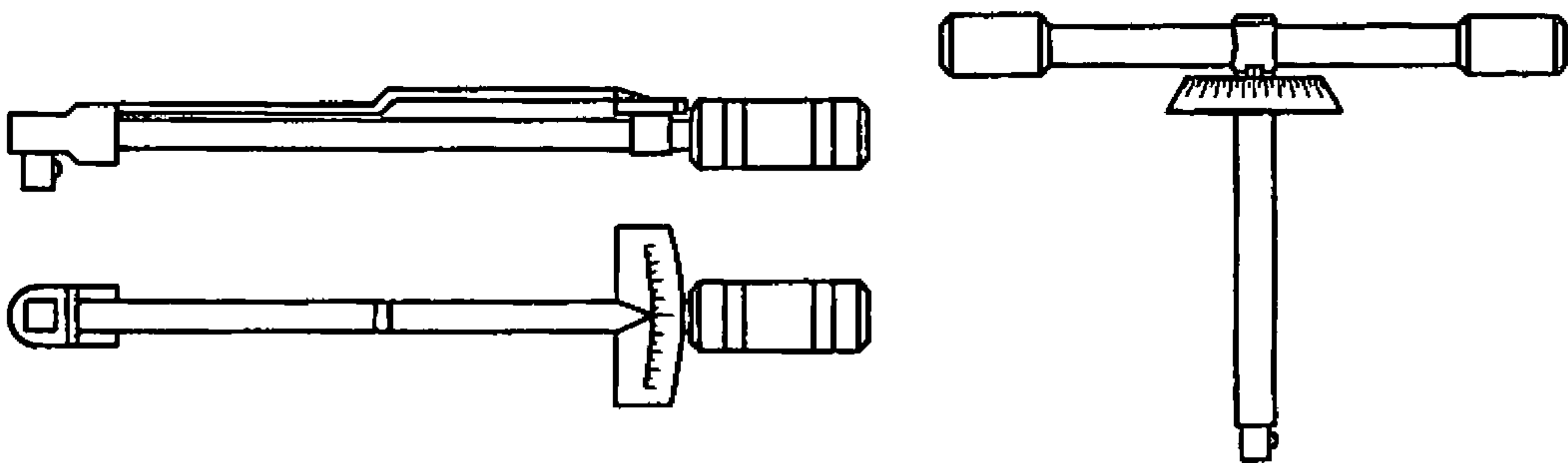
图 A.1 A 型:指针型扭力扳手
