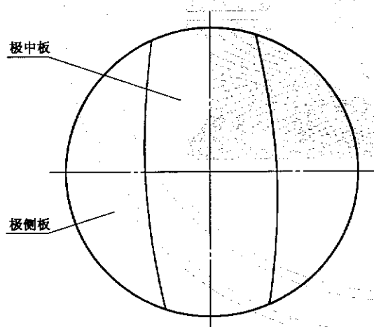
图 11 桔瓣式球罐极带板
