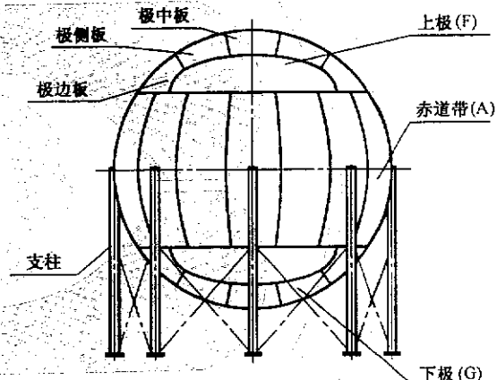
图 6 混合式三带球罐
