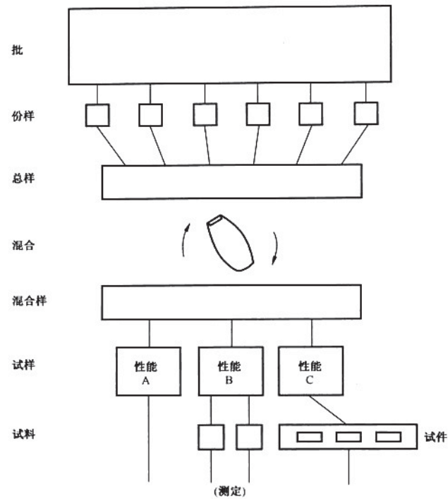
图 1 取样流程
