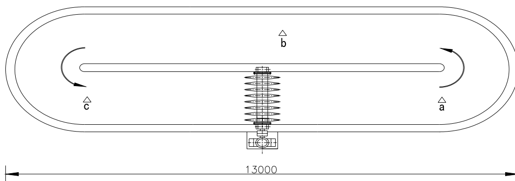
图 1 转盘曝气装置测试采样点布置示意图
