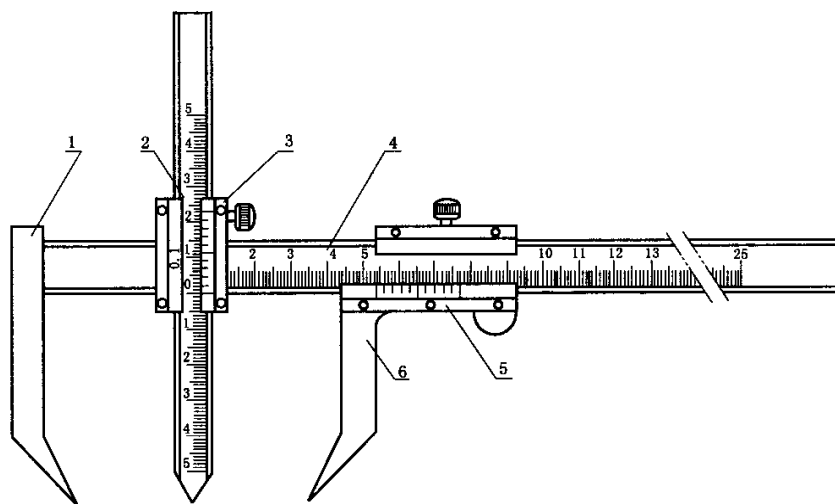
图 4 I 型三脚平行规示意图
