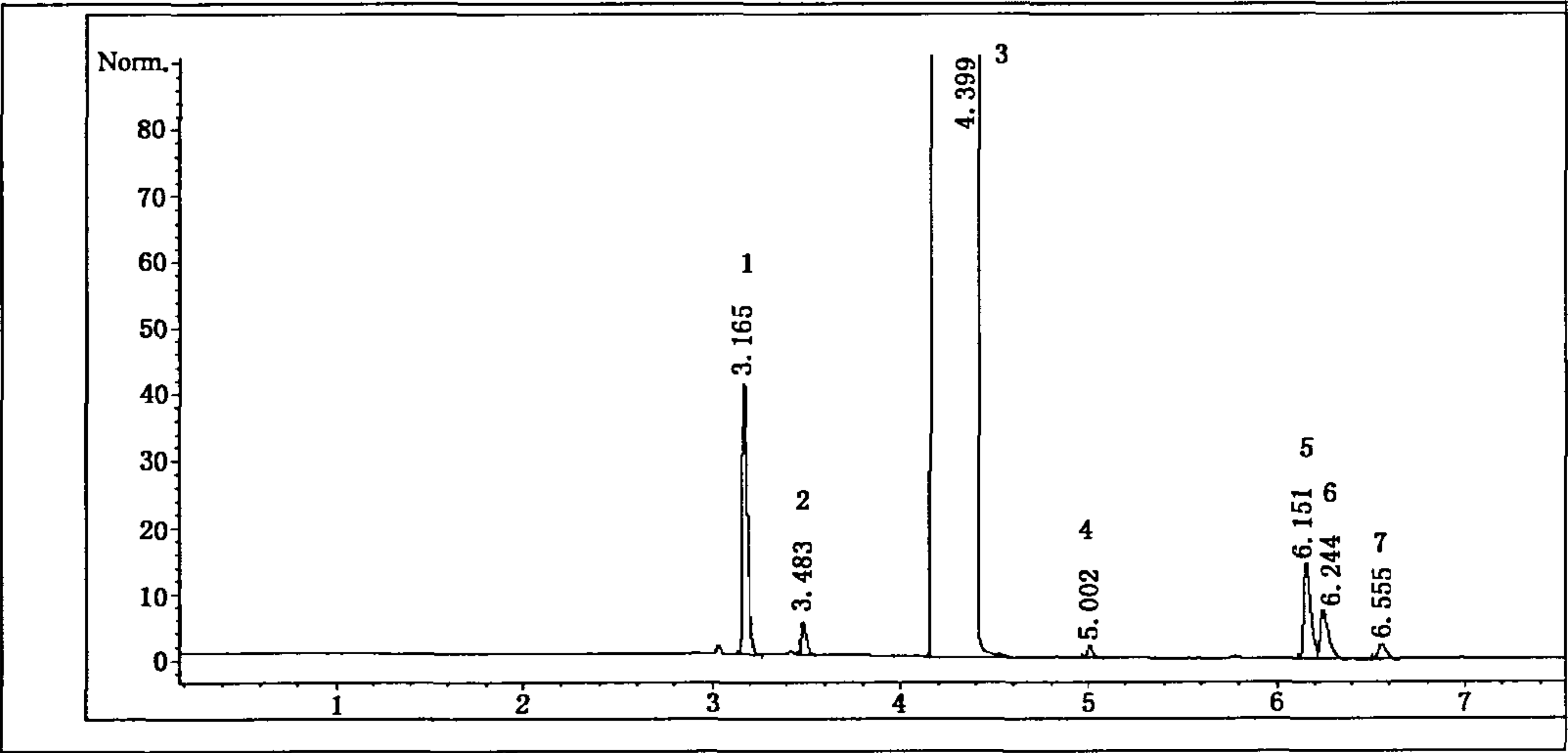
图 A.1 乙酸甲酯的典型色谱图(柱温 40℃)
