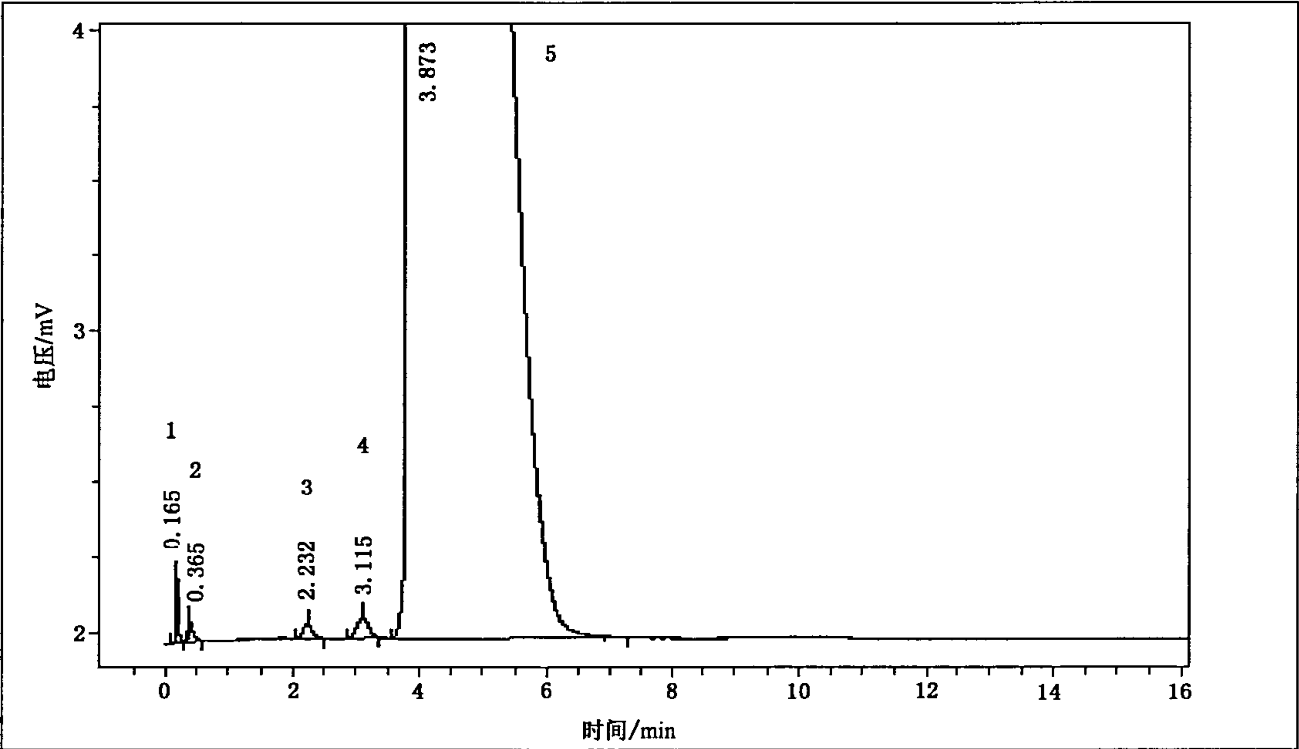
图 A. 10 乙酸异丙酯的典型色谱图
