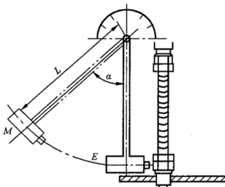
a) 耐冲击性试验装置
