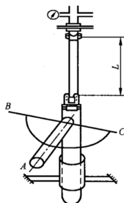
图 4 扭曲试验
