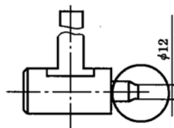
b) 重锤形状及尺寸
