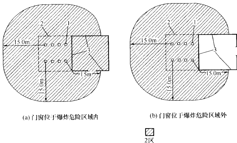
图 A.0.6 无释放源的建筑与通风良好且有二级释放源的建筑相邻,当采用不燃烧体实体墙隔开时,
