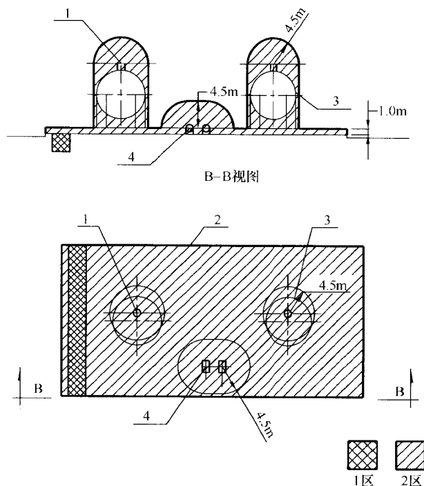
图 A.0.3 地上液化石油气储罐组爆炸危险区域等级和范围划分图
