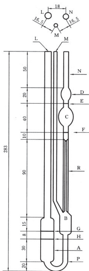
A—低部贮球,外径 26 mm;B—悬浮水平球;C—计时球,容积 3.0 mL( \pm 5\% ); D—上部贮球;E、F—计时标线;G、H—充装标线;L—架置管,外径 11 mm; M—下部出口管,外径 6 mm;N—上部出口管,外径 7 mm;P—连接管,内径 6.0 mm( \pm 5\% );R—工作毛细管,内径 0.50 mm( \pm 2\% )
