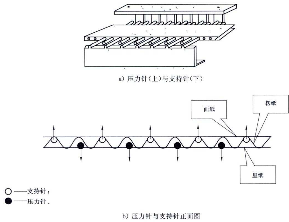
图 2 插针示意图
