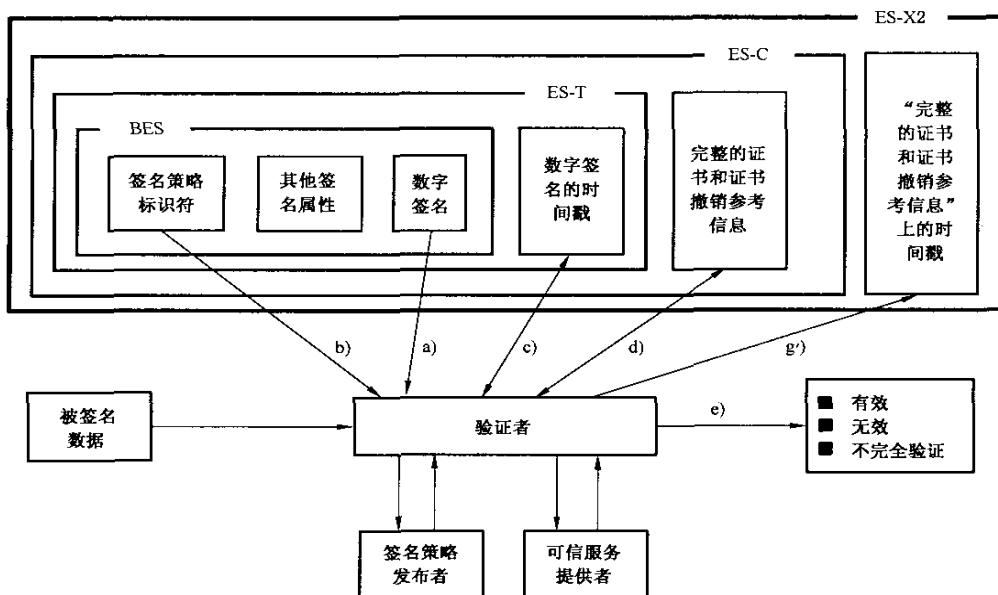
图 14 验证者创建 ES-X2
