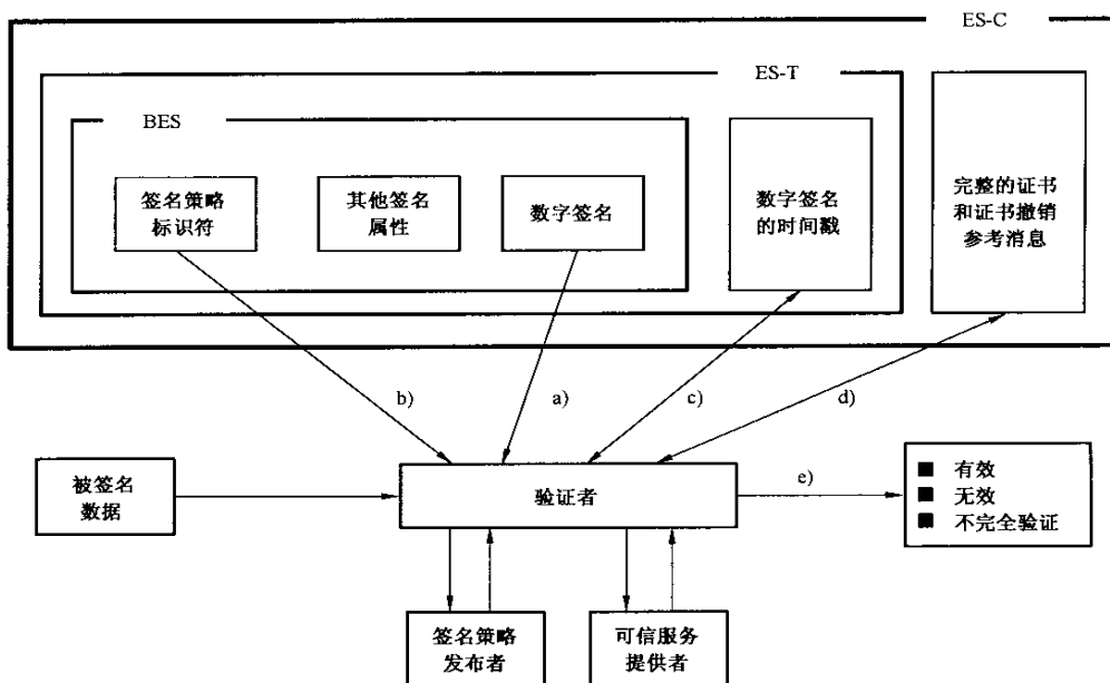
图 11 ES-C 的验证过程
