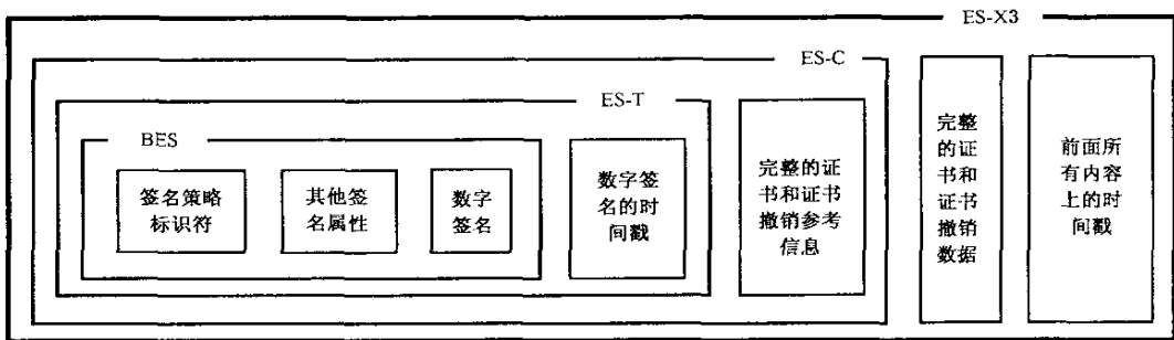
图 8 ES-X3 组成结构
