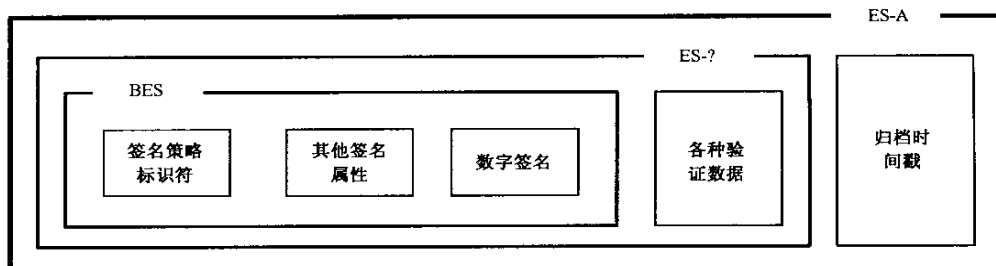
图 10 ES-A 基本结构
