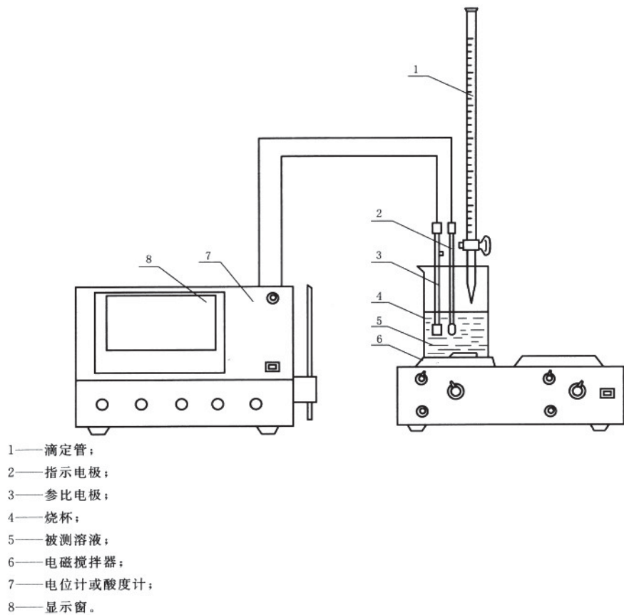
图 1 电位滴定测定装置
