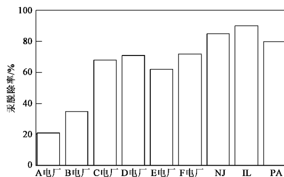
图中 NJ、IL、PA 分别是 New Jersey、Illinois、Pennsylvania 的缩写 图 1 我国燃煤电厂和美国一些州的燃煤电厂汞的脱除率比较
