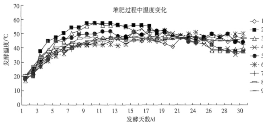
图 2 堆肥过程中的温度变化
