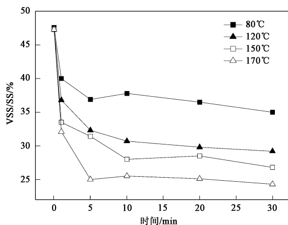
图 2 VSS/SS 变化规律
