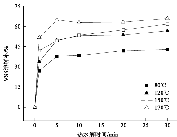
图 1 VSS 溶解率变化规律
