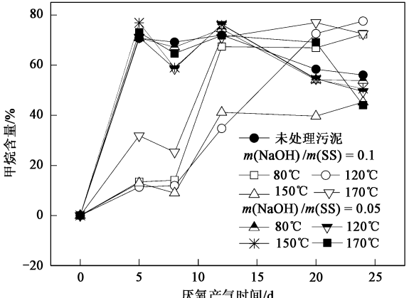
图 10 不同碱添加量下的甲烷含量 Fig. 10 Methane content at different alkali addition dose
