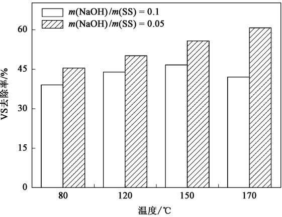
图 9 不同碱添加量下的 VS 去除率 Fig. 9 VS removal ratio at different alkali addition dose
