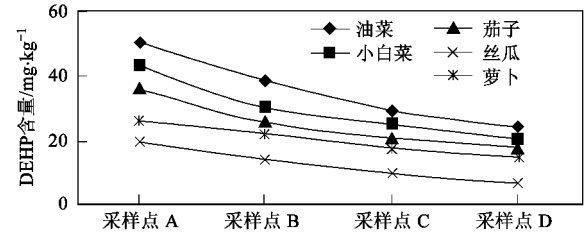
图3 不同采样点蔬菜可食用部分 DEHP 含量 Fig.3 DEHP concentrations in different sampling points of vegetables
