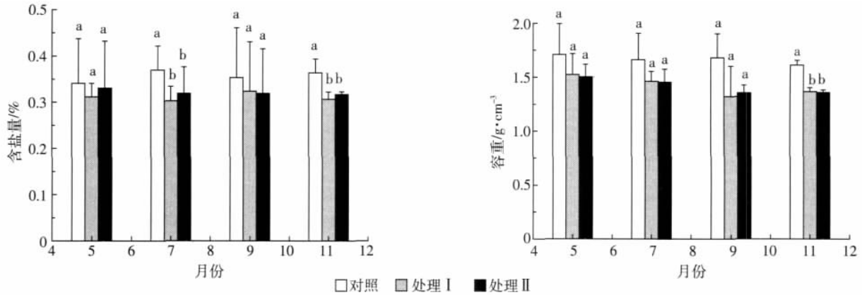
图 2 不同改良模式土壤含盐量和容重的变化趋势
