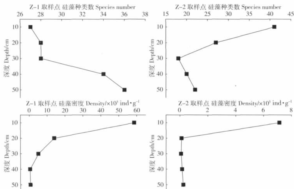
图 3 Z-1、Z-2 钻孔沉积物中硅藻种类数与密度的垂直变化
