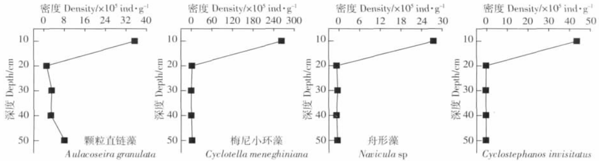
图 5 Z-2 钻孔沉积物中优势种密度的垂直变化
