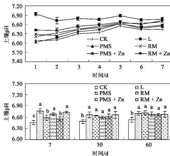
图 1 不同时期各处理的土壤 pH 变化
