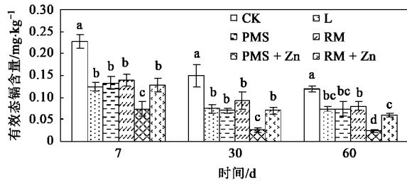
图2 不同时期各处理的土壤有效态镉含量变化 Fig. 2 Changes of soil available Cd content in each treatment in different periods
