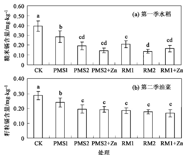
图 5 不同处理水稻糙米、油菜籽粒镉含量变化
