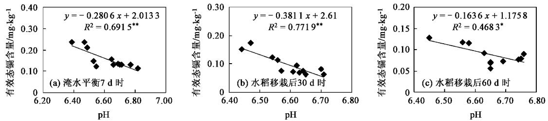
图3 不同时期各处理土壤有效态镉含量与 pH 的相关关系 Fig. 3 Regression analysis on available Cd in soil and soil pH value in each treatment in different periods
