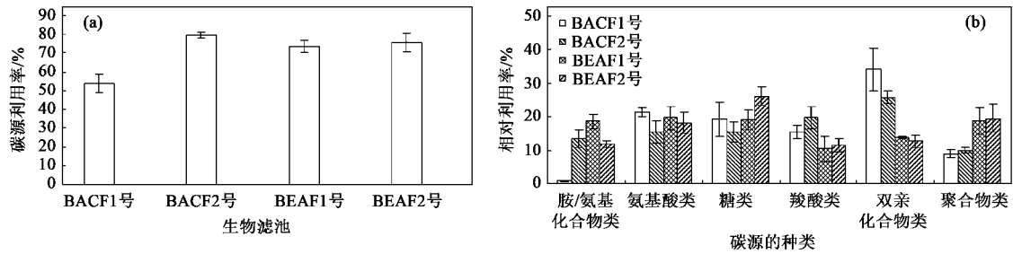
图3 不同生物滤池中微生物群落对碳源的利用情况
