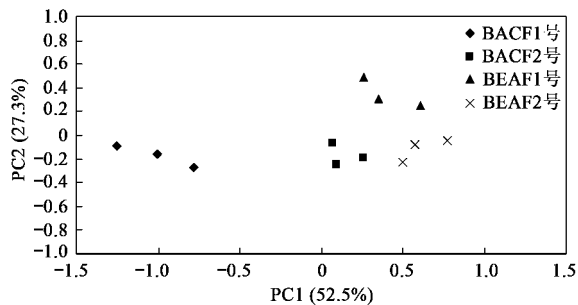
图4 各生物滤池中微生物群落碳源利用谱主成分分析
