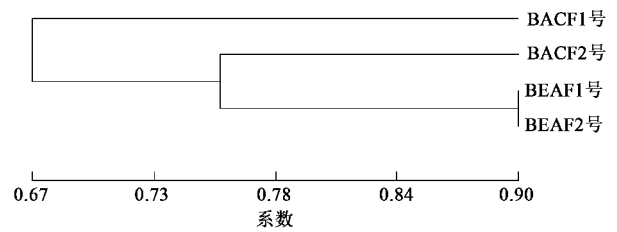
图5 不同生物滤池中微生物群落利用碳源谱的聚类分析
