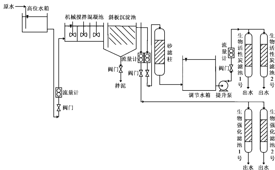
图 1 净水装置示意
