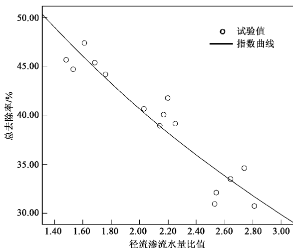
图8 植被缓冲带径流渗流水量比值与总去除率曲线拟合关系
