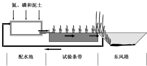
图 3 缓冲带现场试验工艺流程 Fig.3 Process flow chart of buffer strips field test
