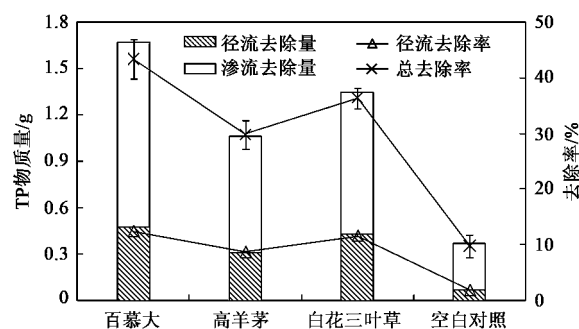
图7 不同植被缓冲带径流渗流TP去除量及其去除率
