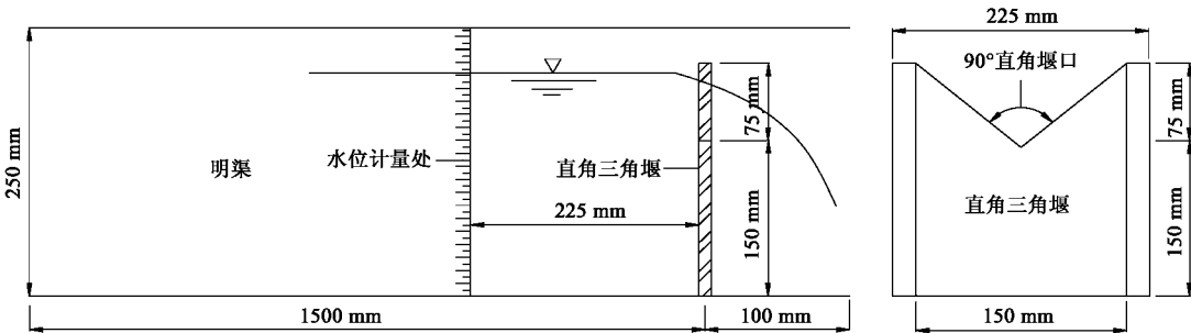
图2 直角三角堰装置示意
