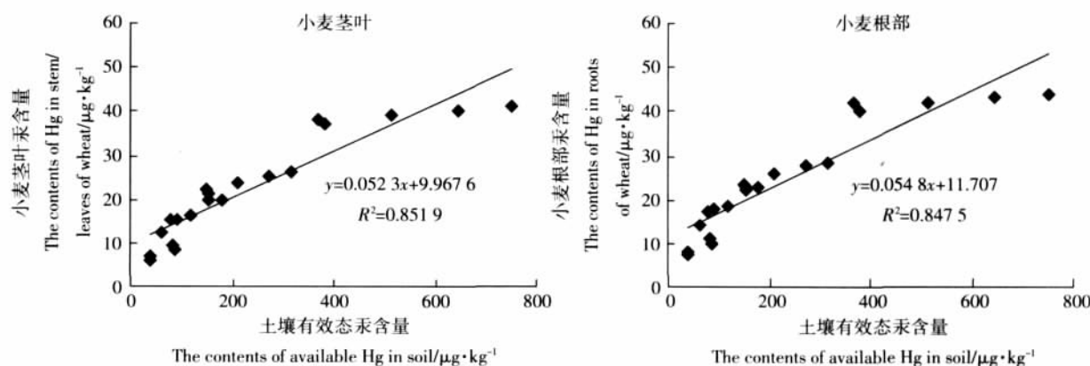
图2 土壤有效态汞含量与小麦茎叶和根部汞含量之间的关系
