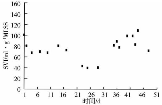
图 4 MBR 中污泥 SV 随时间的变化
