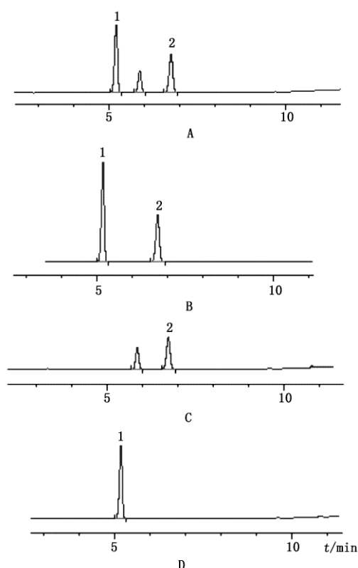
图1 对照品 A 样品 B 阴性样品 C 阴性样品 D 气相色谱图 Fig 1 GC chromatograms reference of substance (A) sample (B) negative sample without Menthol (C) negative sample without Borneol (D)
