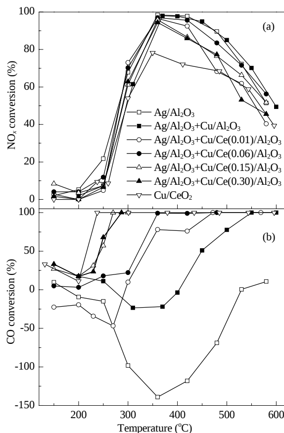
图5 不同催化剂体系中乙醇选择性还原 \text{NO}_x 中 \text{NO}_x 及CO转化率随反应温度的变化
