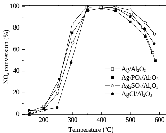
图 6 各种负载型难溶性银化合物催化剂催化乙醇选择性还原 NO x 的活性
