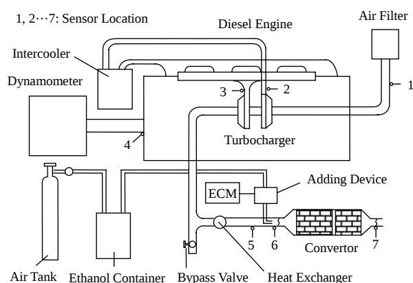
图 8 \text{NO}_x 选择性还原台架实验示意图
